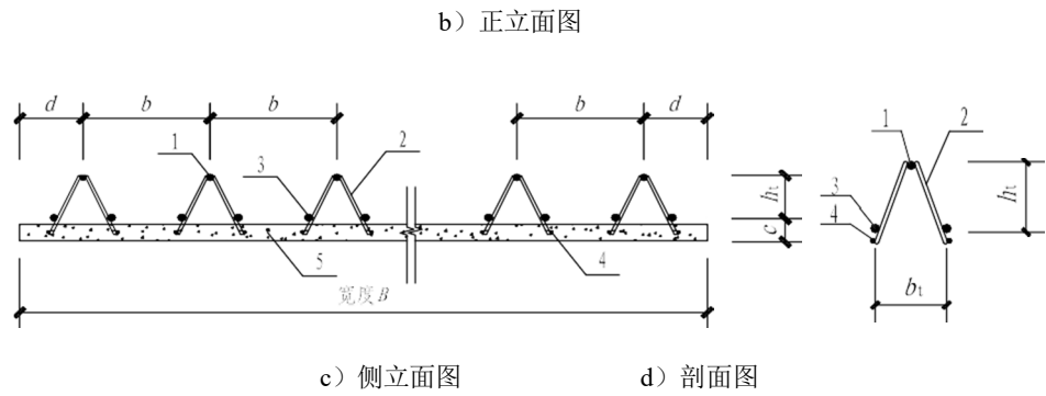
图 4.3.1-1 钢筋桁架板构造示意图一
