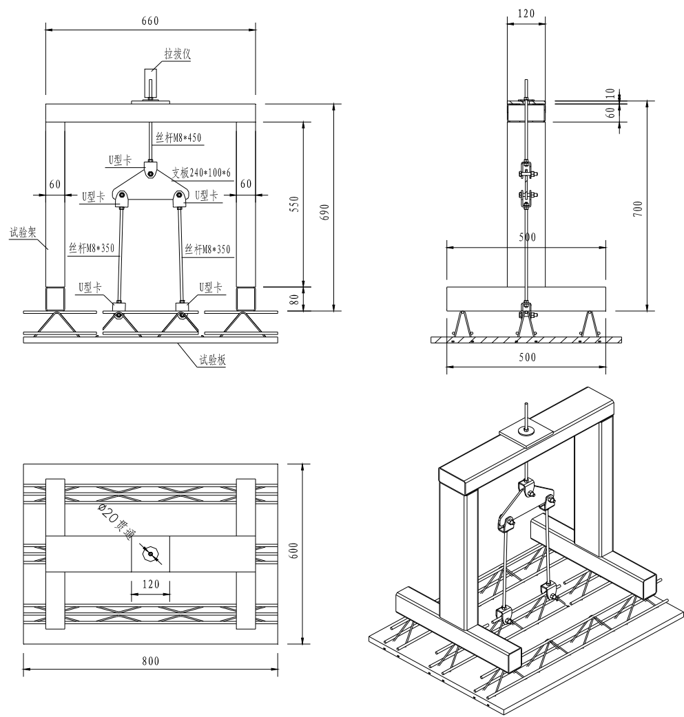
图 B.0.3 抗拉试验装置示意图
