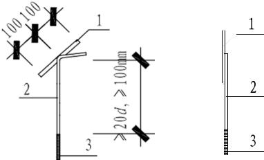
图 B.0.2 钢筋桁架腹杆和弦杆焊点受剪试件
