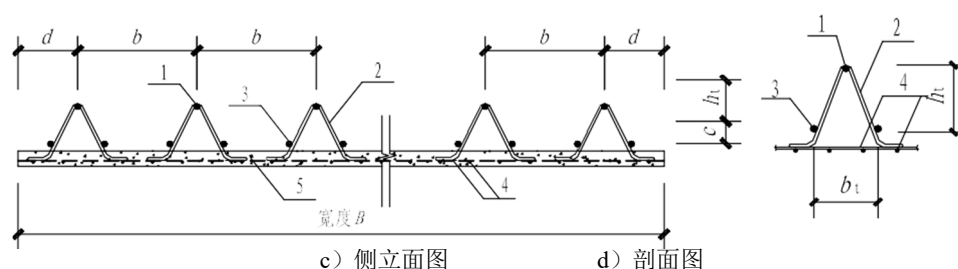
图 4.3.1-2 钢筋桁架板构造示意图二
