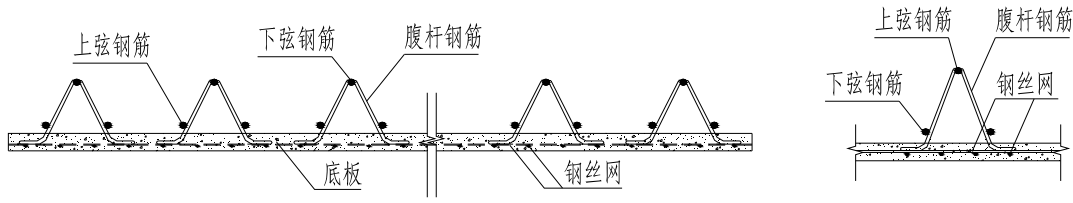
图 1 钢筋桁架板构造示意图一
