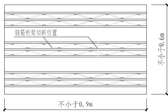
图 D.0.2 钢筋桁架与底板的连接点抗拉试验试件
